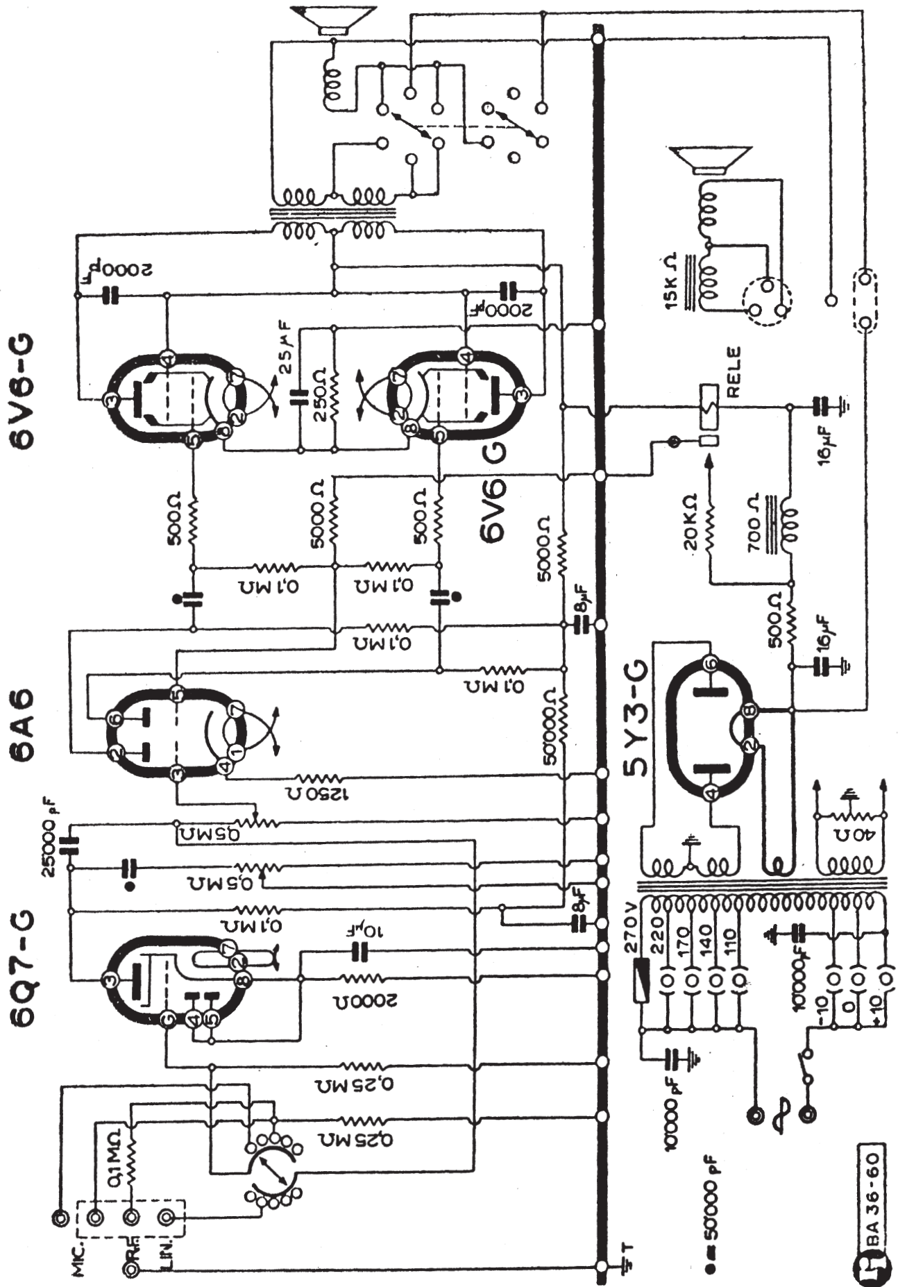
UNDA RADIO - AMPLIFICATORE PORTATILE MOD. « P5/2 »
