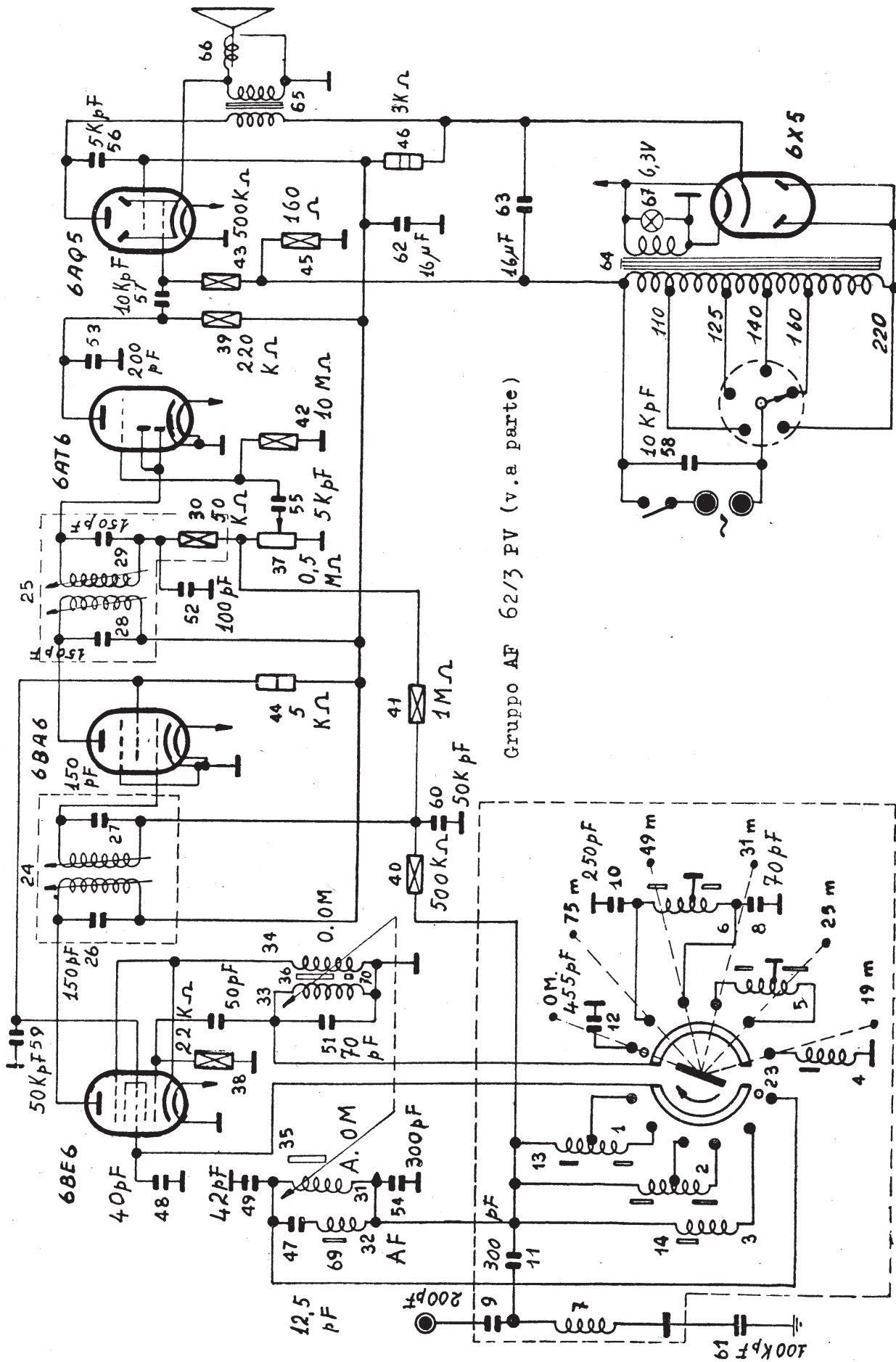
UNDA RADIO - Mod. 56/2. Supereterodina a 6 gamme d'onda: 182-578 m e bande allargate di 19, 25, 31, 49, 75 m. Media frequenza 467 kc. Consumo: 40 watt, cc. 60 mA, ca. 220 mA, ca. 220 mA, Potenza d'uscita 2 watt.
