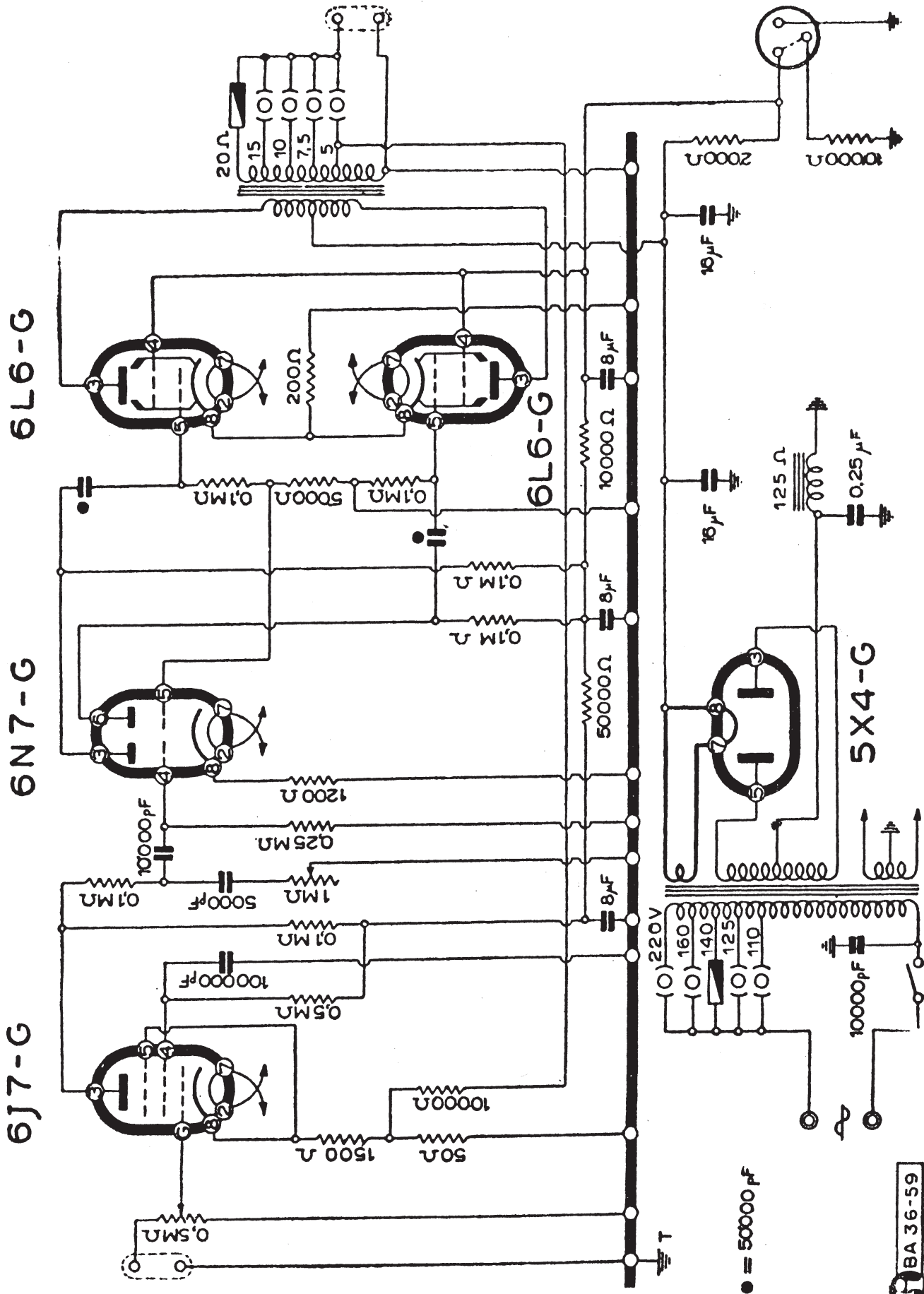
UNDA RADIO - AMPLIFICATORE FISSO MOD. « P5/1 »
