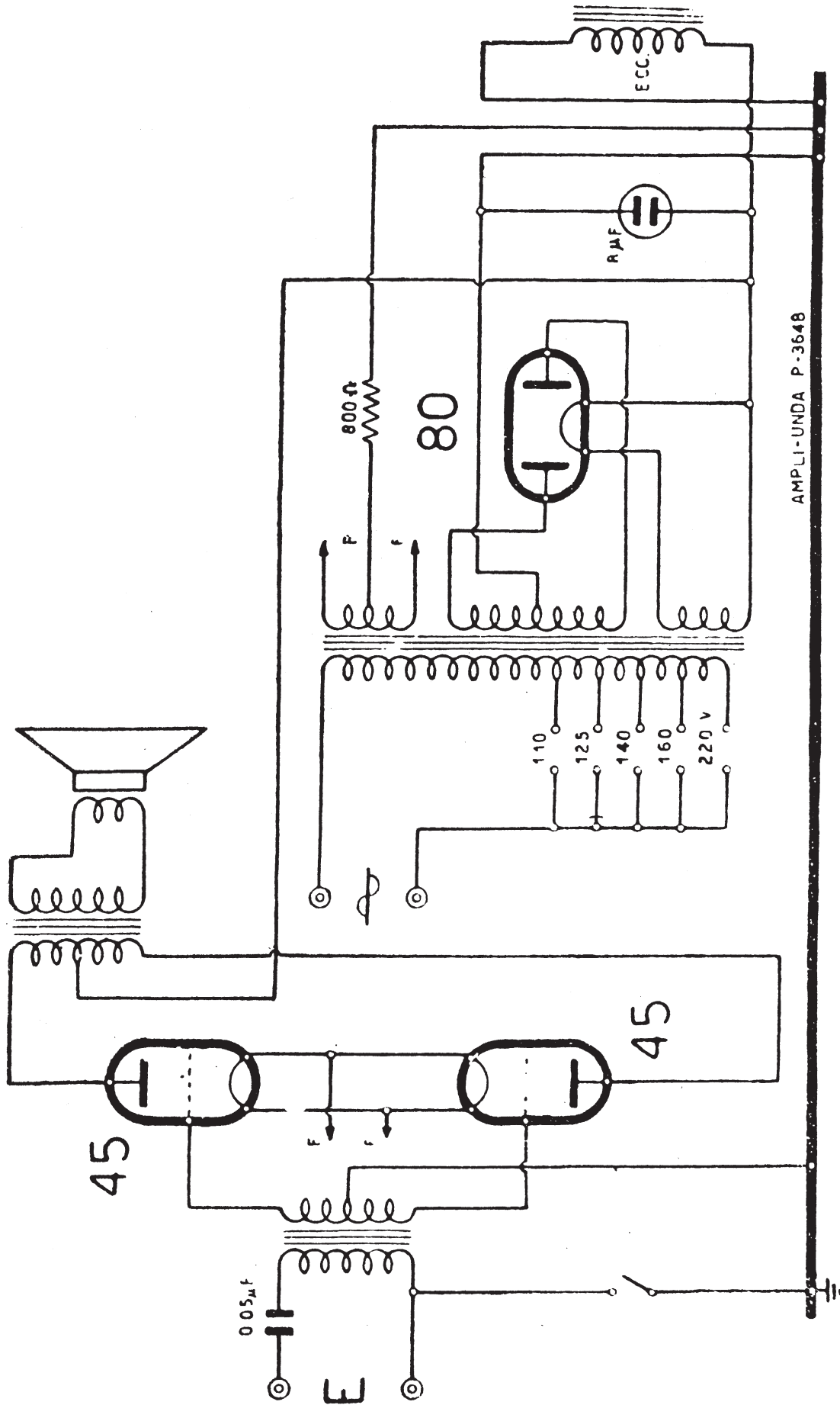
UNDA RADIO - AMPLIFICATORE MOD. « AMPLI UNDA »
