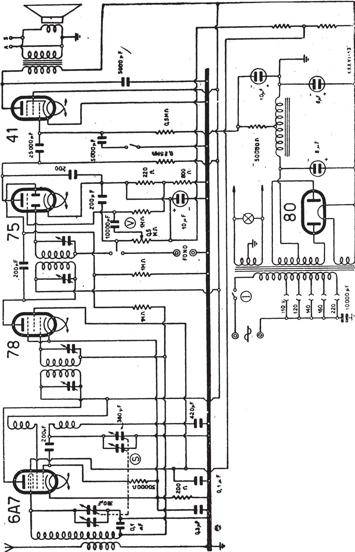
UNDA RADIO - MOD. « BI UNDA 15 »
