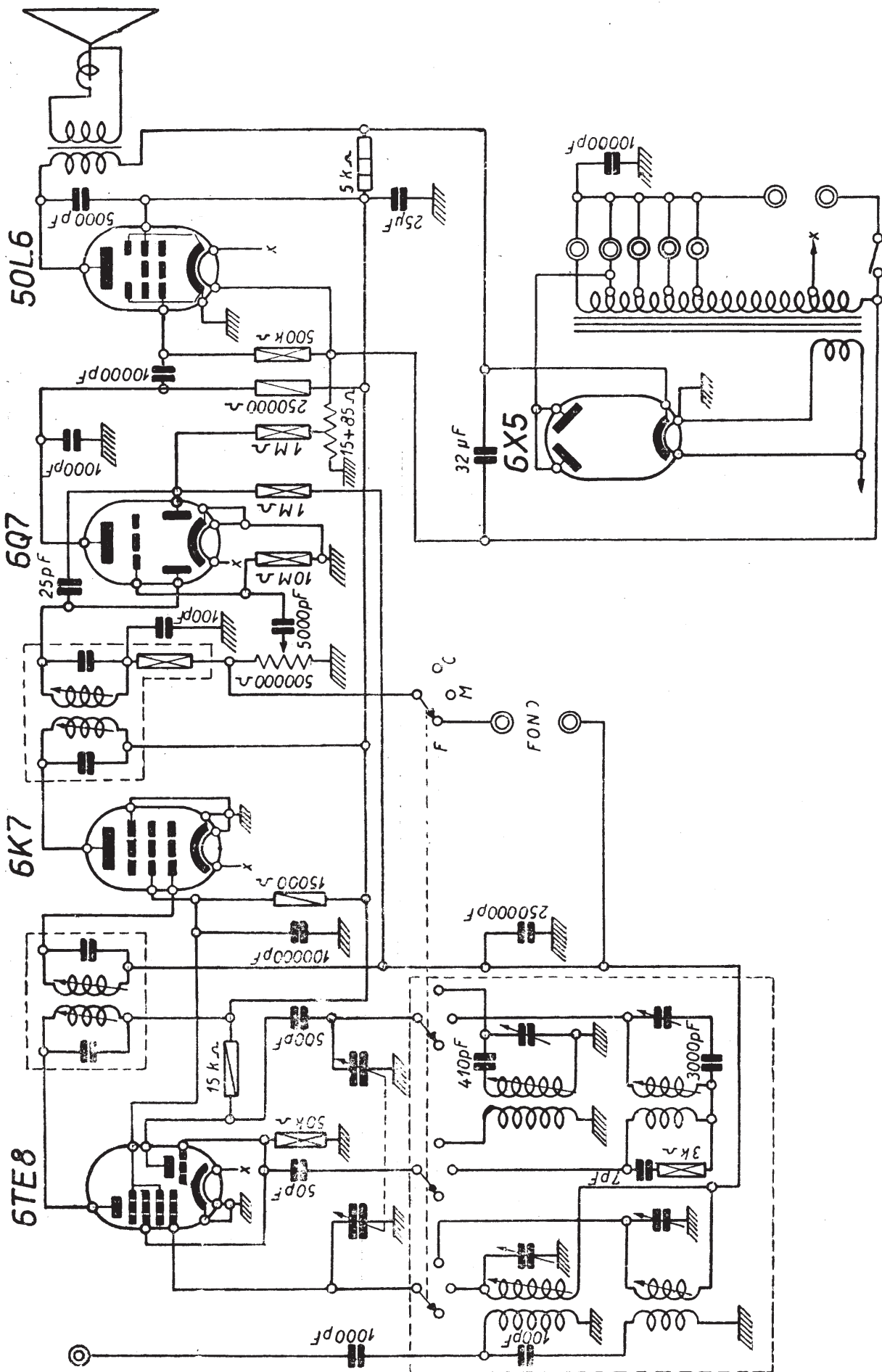
UNDA RADIO - Mod. R 52/1 - Medie e corte. Media frequenza 450 kc/s. Tensioni 6TE8; 105 V pl. ecc., 75 V pl. tr., -1 V griglia. 6K7: 105 V pl., 57 V sch., -1 V griglia. 6Q7: 57 V placca, 50L6: 160 V pl., 175 V catodo. Corrente totale 70 mA.
