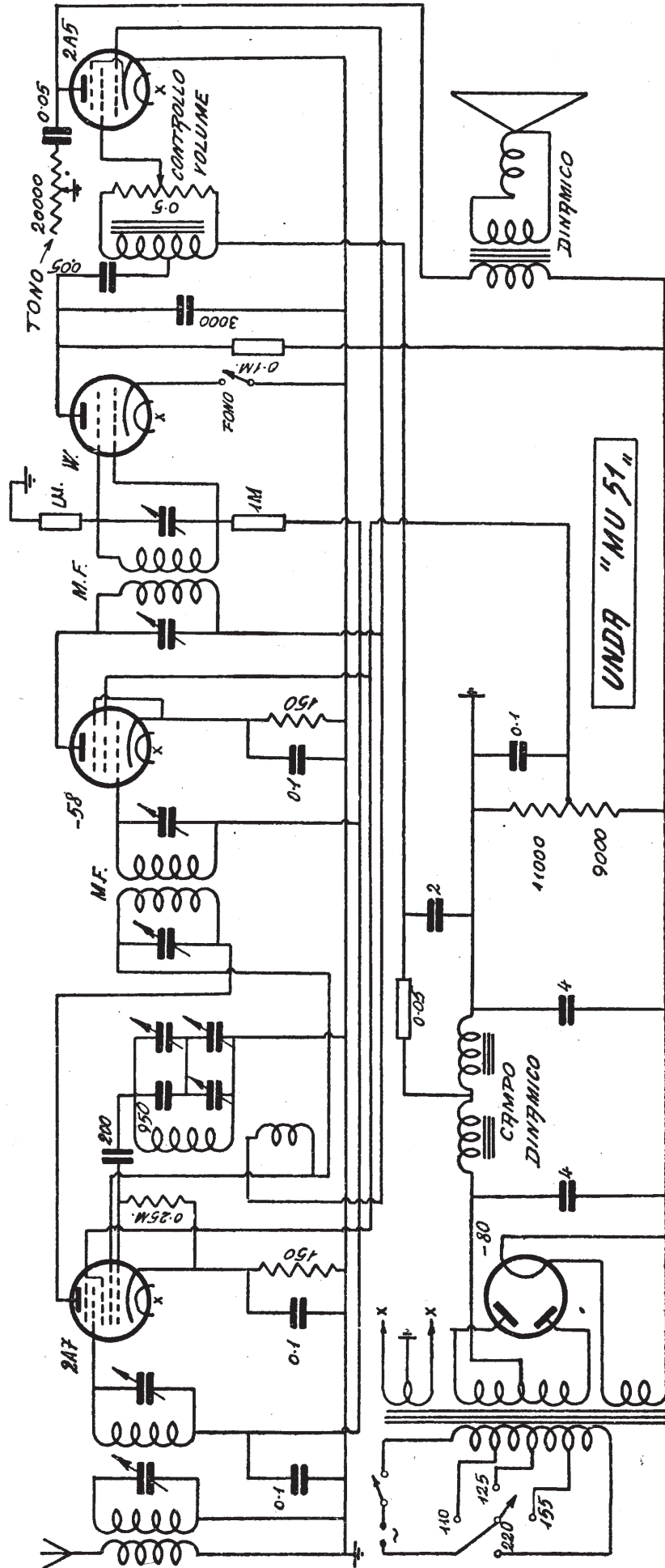
126. — UNDA RADIO. — Modello « M. U. 51 ». - Produzione 1933. - Media frequenza: 175 kc.
