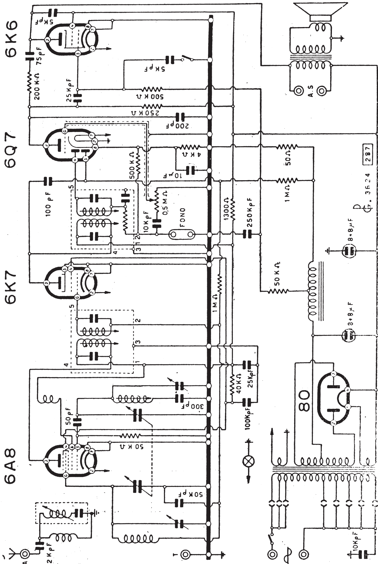
UNDA RADIO - MOD. « MONO UNDA 511 »
