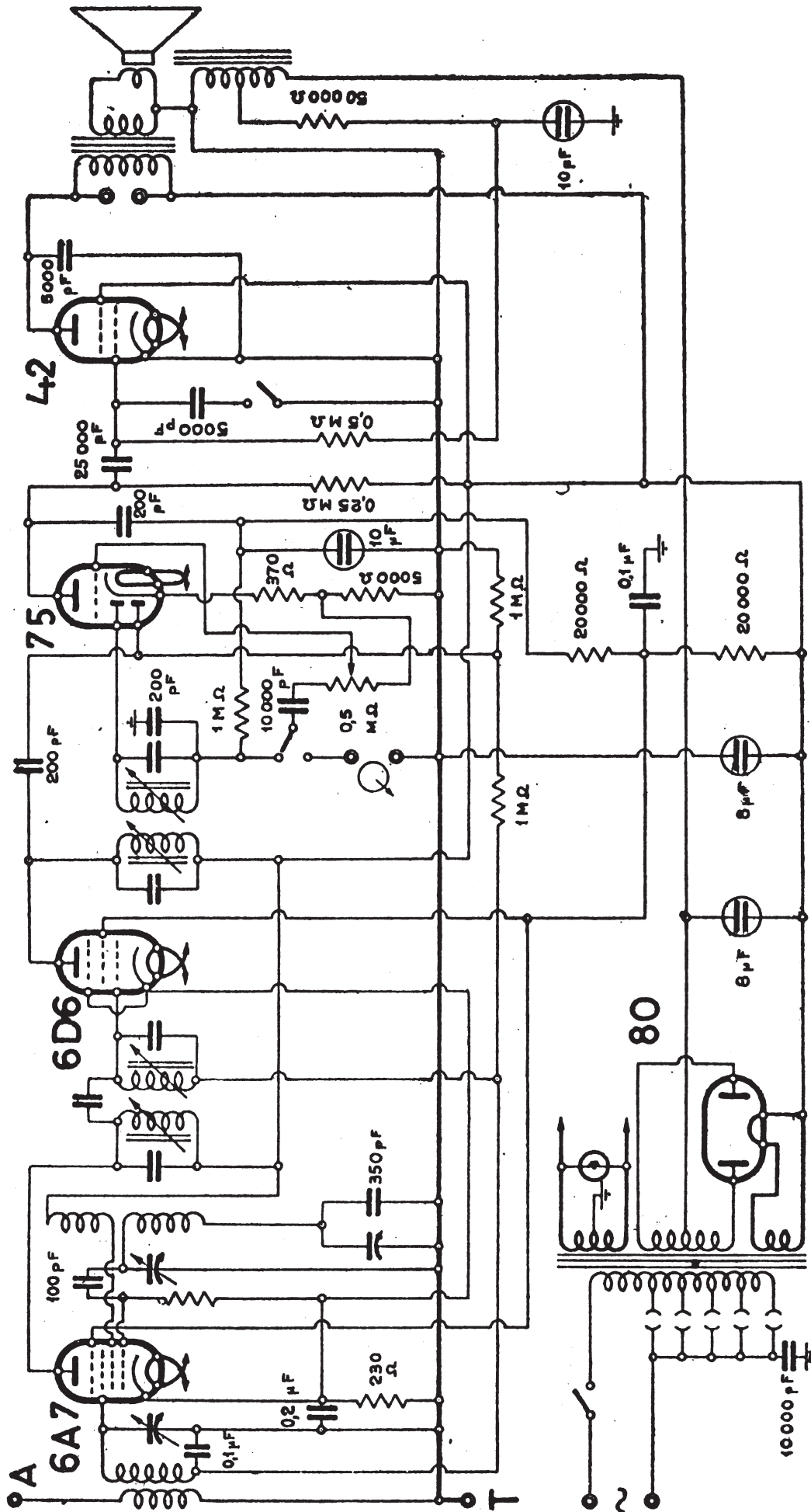
UNDA RADIO - MOD. « MONO UNDA 537 »
