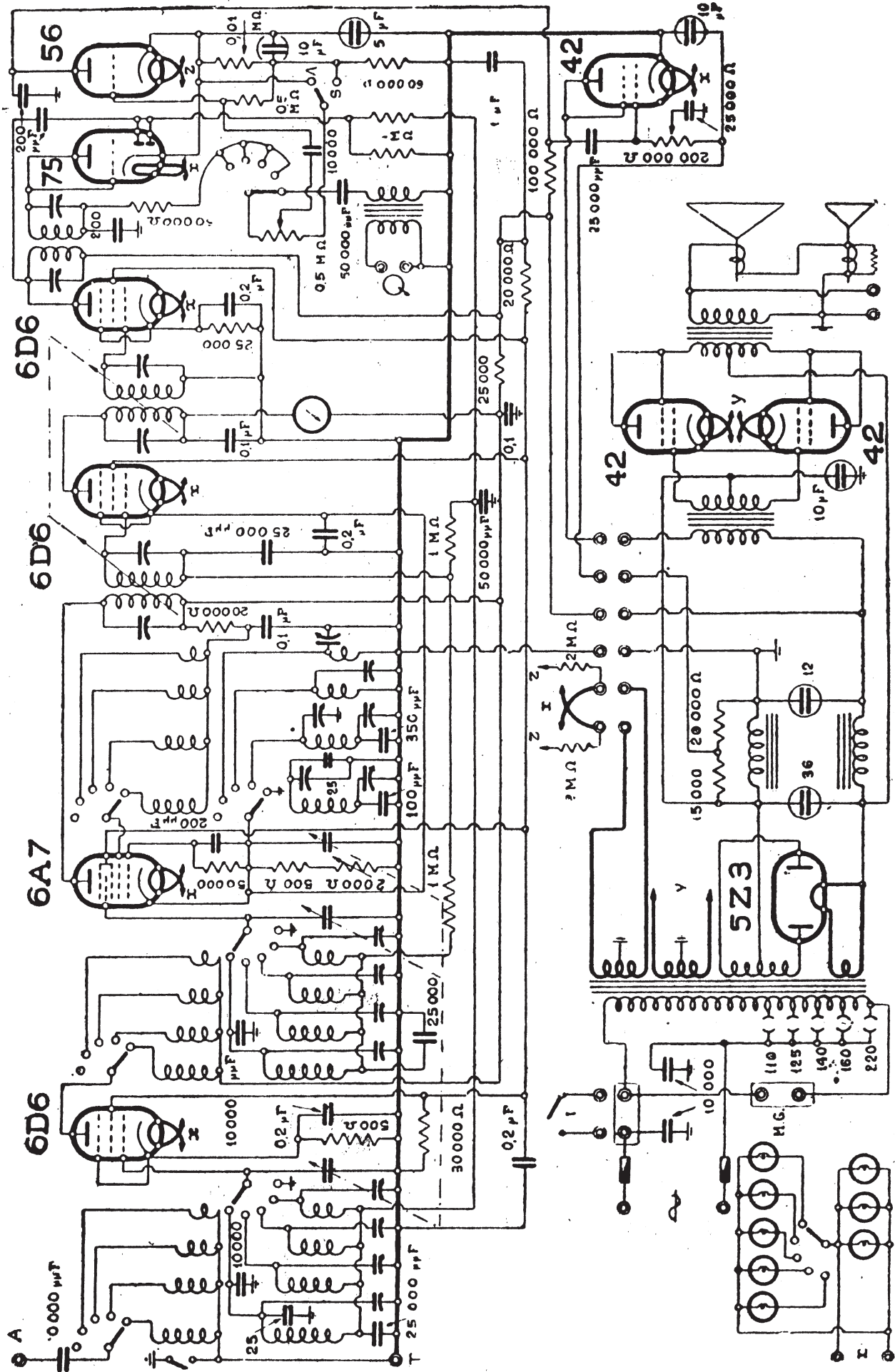
UNDA RADIO - MOD. « QUADRI UNDA 100 »
