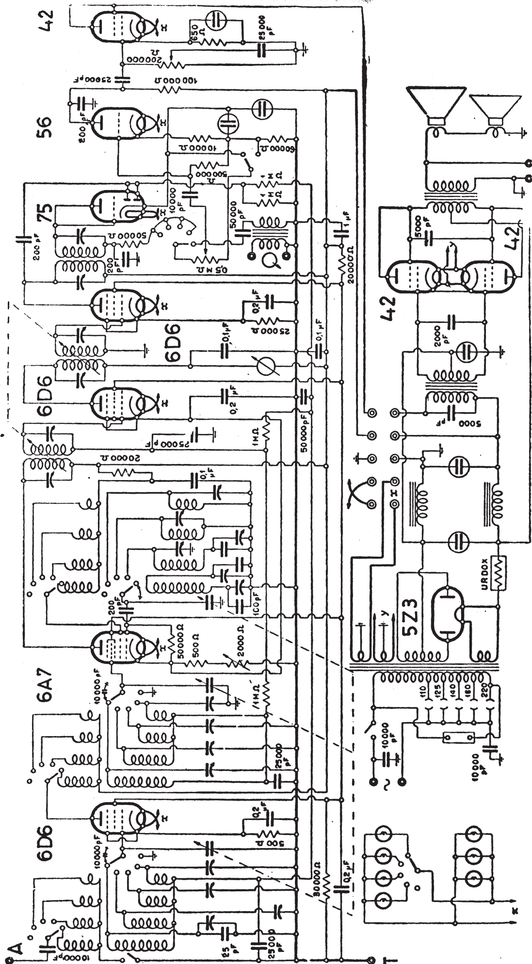
UNDA RADIO - MOD. « QUADRI UNDA 1037 »
