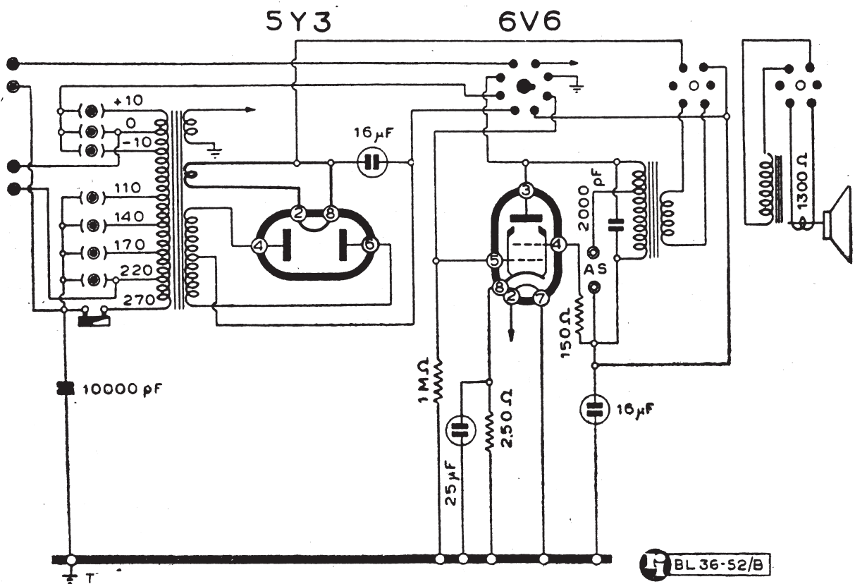
UNDA RADIO - MOD. « QUADRI UNDA 54/1 » PARTE BF E ALIM.
