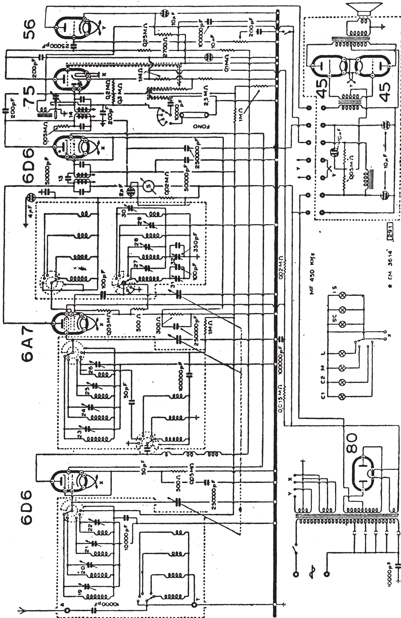
UNDA RADIO - MOD. « QUADRI UNDA 837 »
