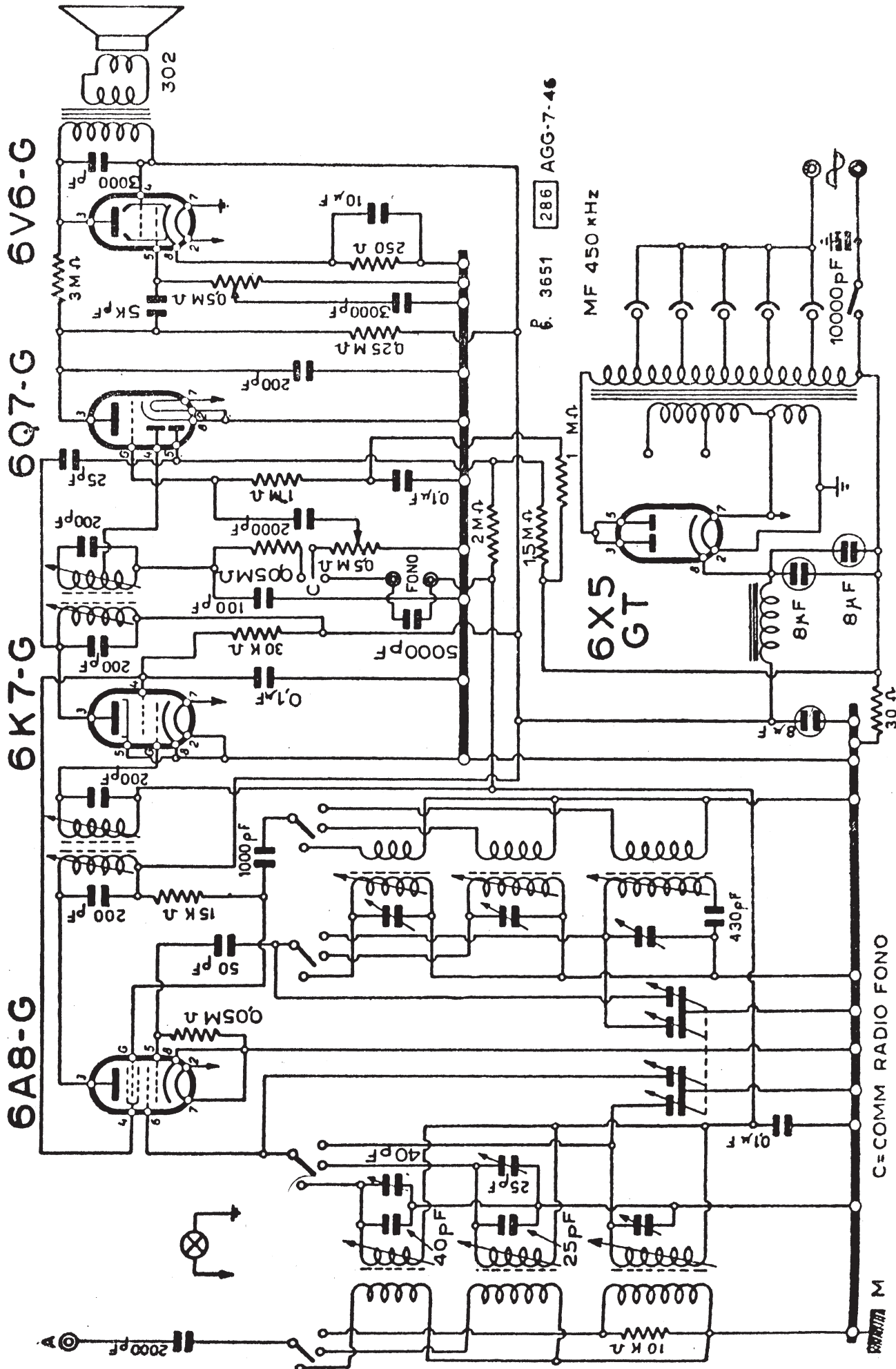
UNDA RADIO - MOD. « TRI UNDA R 53/4 »
