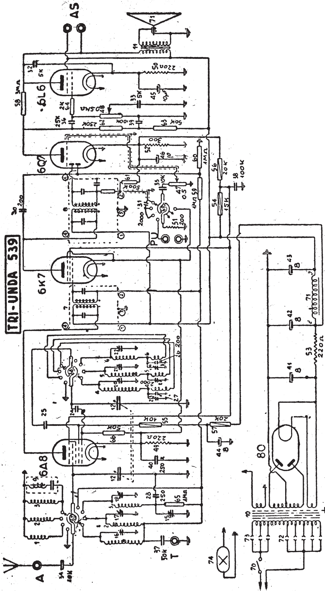
UNDA RADIO. — Modello Tri-Unda 539. — Produzione 1938-39. — Gamme: cc. (15-30). c. (30-80), m. (206,5-600). — Potenza d'uscita: 5,5 W. — Media frequenza: 450 kHz.
